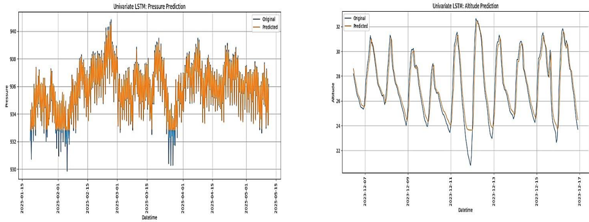
Gambar 3. Grafik data asli dan hasil prediksi LSTM univariat
